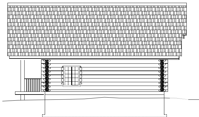
RIGHT ELEVATION
